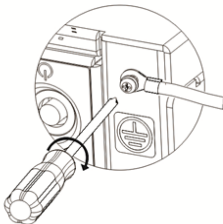
图4-22 安装接地线示意图
