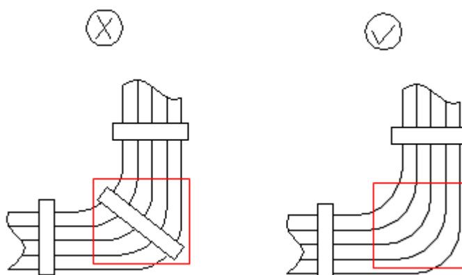
图4-18 线缆捆扎示意图（三）
