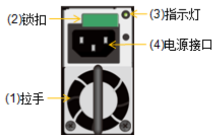
图3-6 SPU 电源模块正视图
