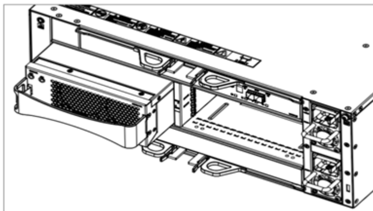
图6-8 安装/拆卸 DSU2624 风扇模块示意图
