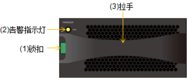
图3-15 DSU2624 风扇模块正视图
