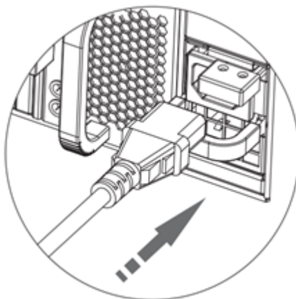
图4-25 安装电源线示意图 (二)
