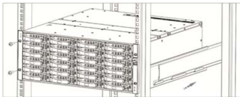
图4-12 安装 SPU 示意图
