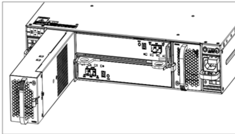
图6-7 安装/拆卸 DSU2625 风扇模块示意图
