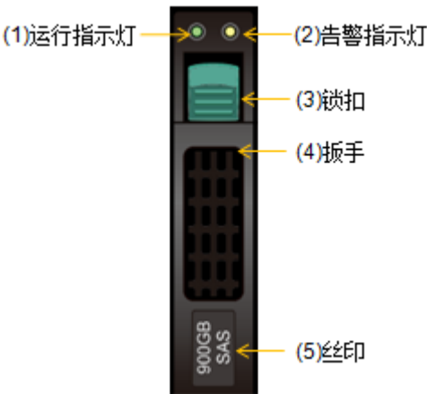
图3-17 2.5 英寸磁盘模块前面板
