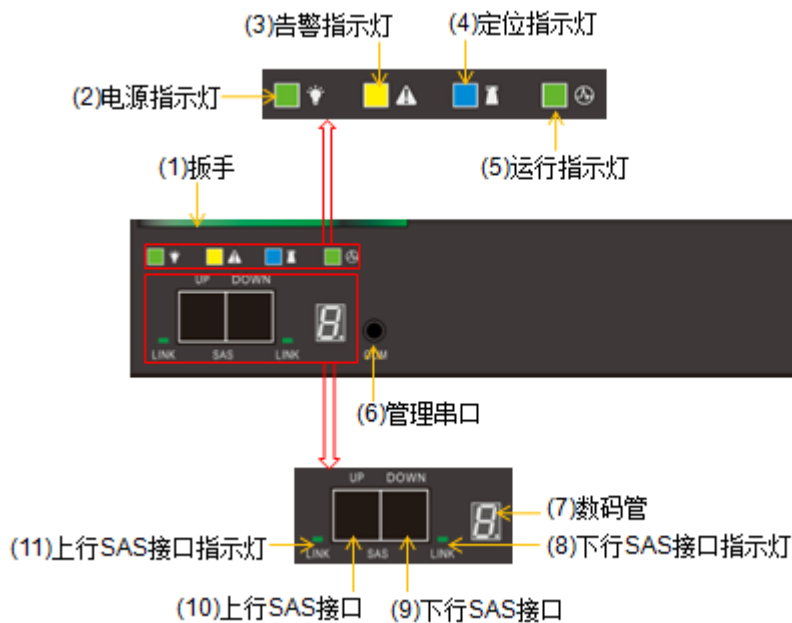
图3-9 DSU2625 的 EP 正视图
