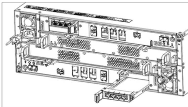
图6-4 安装/拆卸 IO 插卡模块示意图
