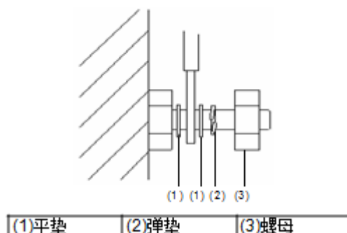
图4-15 固定线缆端子示意图
