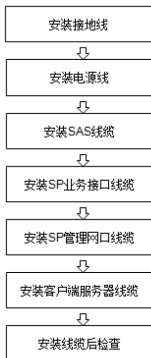
图4-19 线缆安装流程示意图
