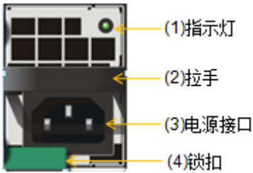
图3-11 DSU2625 电源模块正视图
