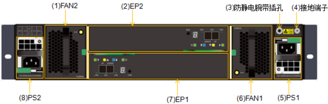
图3-8 DSU2625 后正视图
