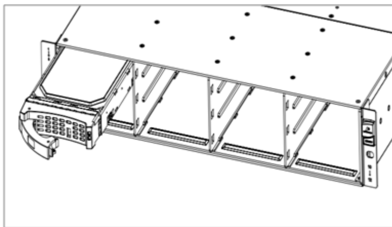
图6-15 安装 3.5 英寸磁盘模块示意图
