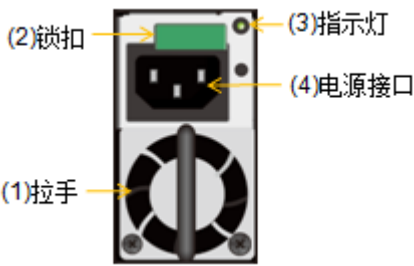
图3-16 DSU2624 电源模块正视图
