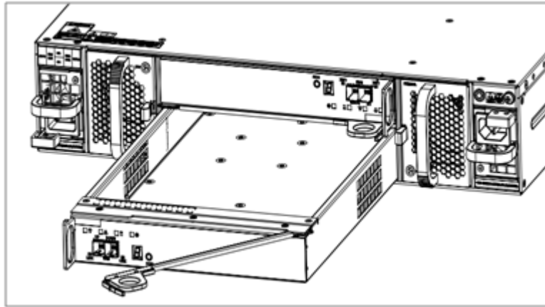
图6-5 安装/拆卸 DSU2625 EP 示意图
