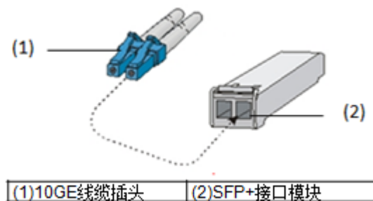
图4-35 10GE 线缆和接口示意图
