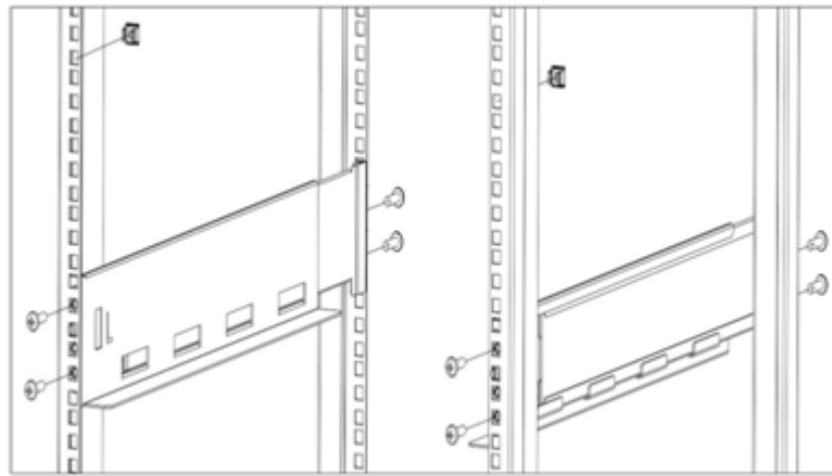
图4-10 安装浮动螺母示意图
