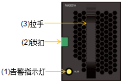
图3-10 DSU2625 风扇模块正视图
