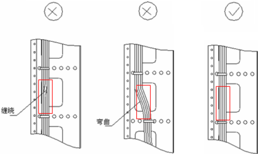
图4-16 线缆捆扎示意图（一）
