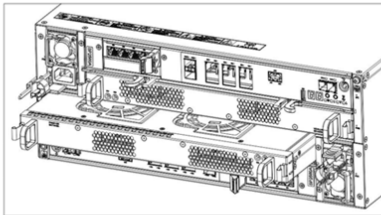
图6-2 安装/拆卸 SPU 风扇模块+电池模块示意图
