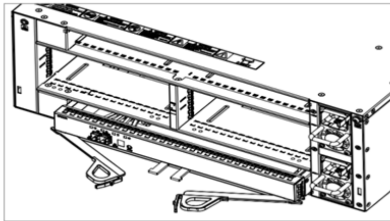
图6-6 安装/拆卸 DSU2624 EP 示意图
