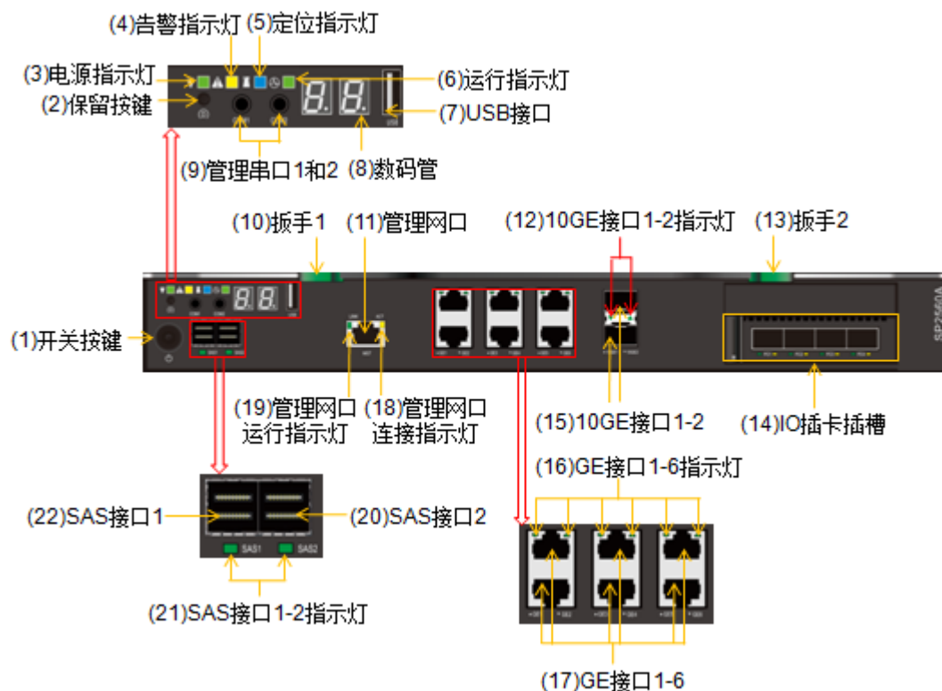
图3-3 SP 正视图
