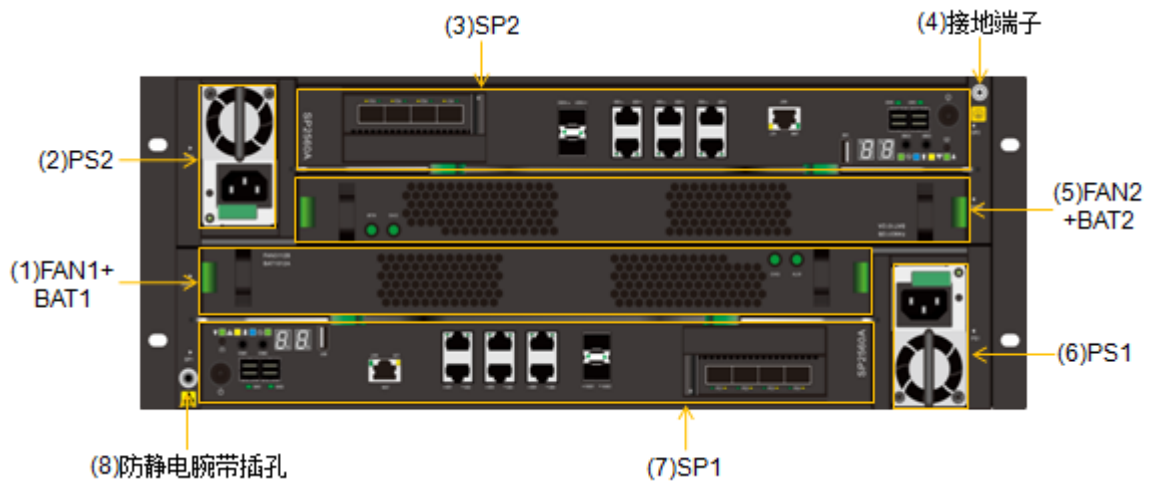
图3-2 SPU 后正视图
