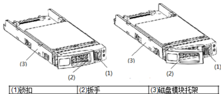
图6-10 2.5 英寸磁盘模块示意图
