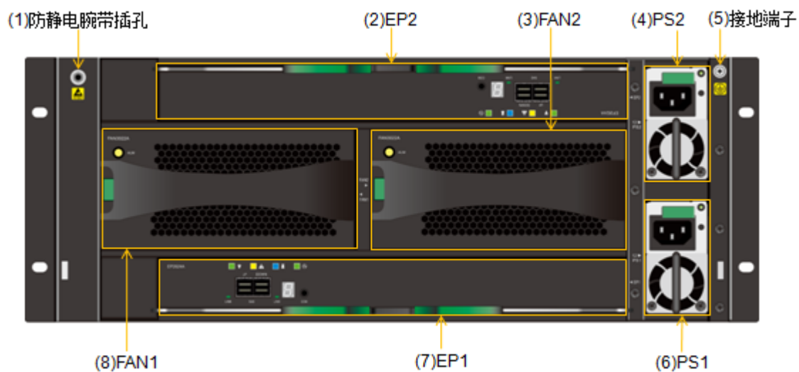
图3-13 DSU2624 后正视图
