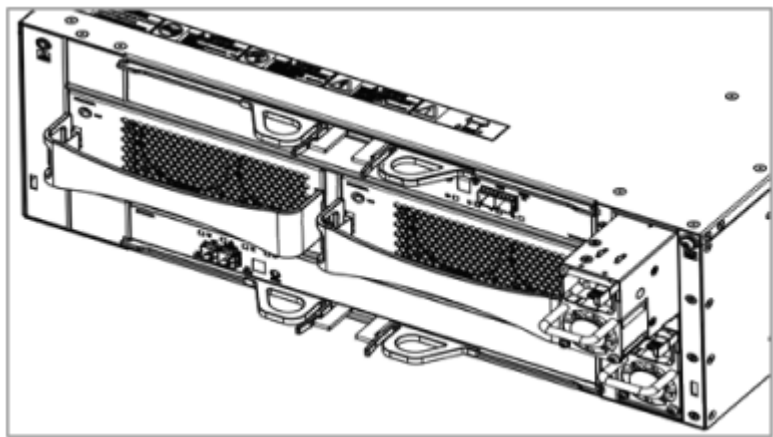
图6-9 安装/拆卸 DSU2624 电源模块示意图
