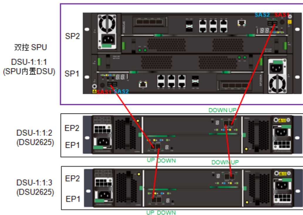
图4-31 SAS 线缆安装示意图
