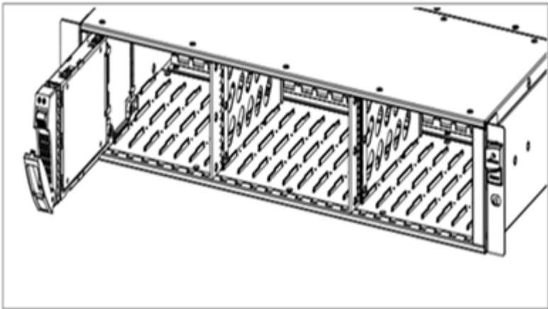
图6-12 安装 2.5 英寸磁盘模块示意图（二）
