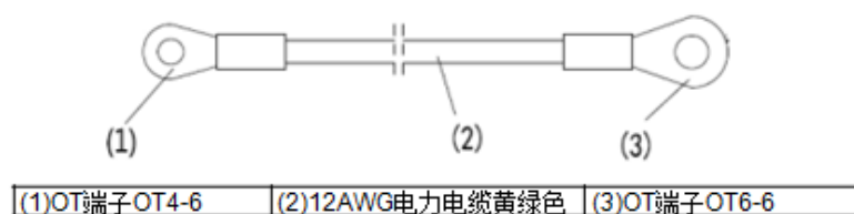
图4-20 接地线示意图
