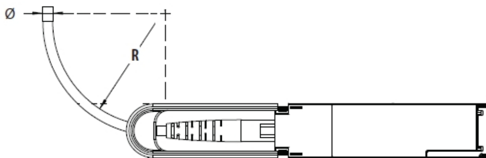
图4-30 AOC 光缆弯曲半径示意图
